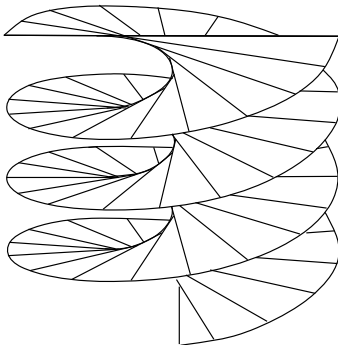
Fig. 13.1 A helicoid
